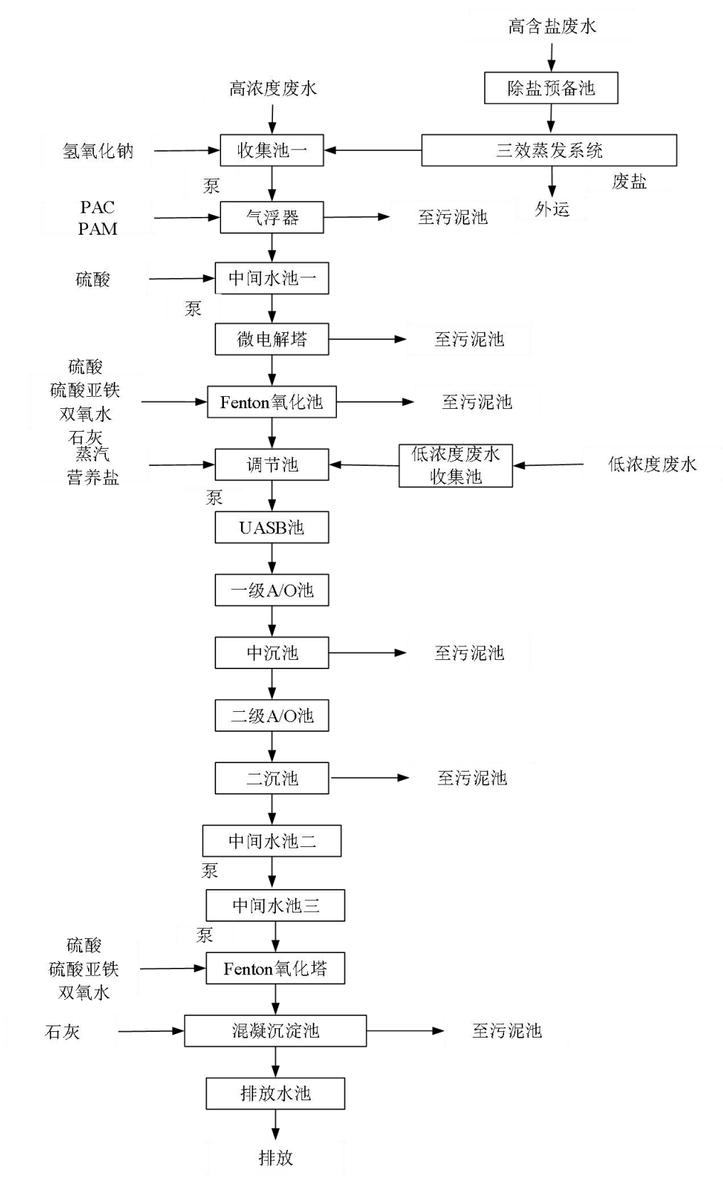
图 4.3-27 废水零排放工艺流程图
