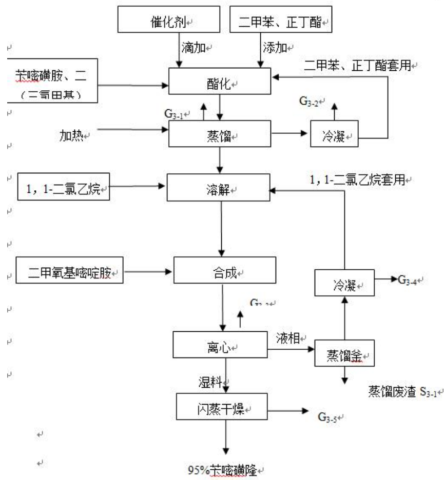
图 4.3-7 苄嘧磺隆生产工艺流程框图
