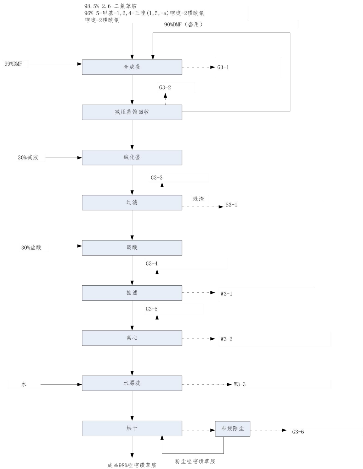
图 4.3-11 唑啉磺草胺生产工艺流程图
