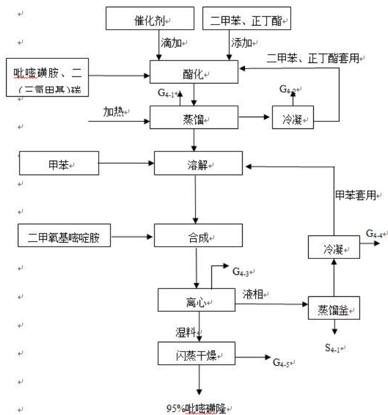
图 4.3-8 吡嘧磺隆生产工艺流程框图
