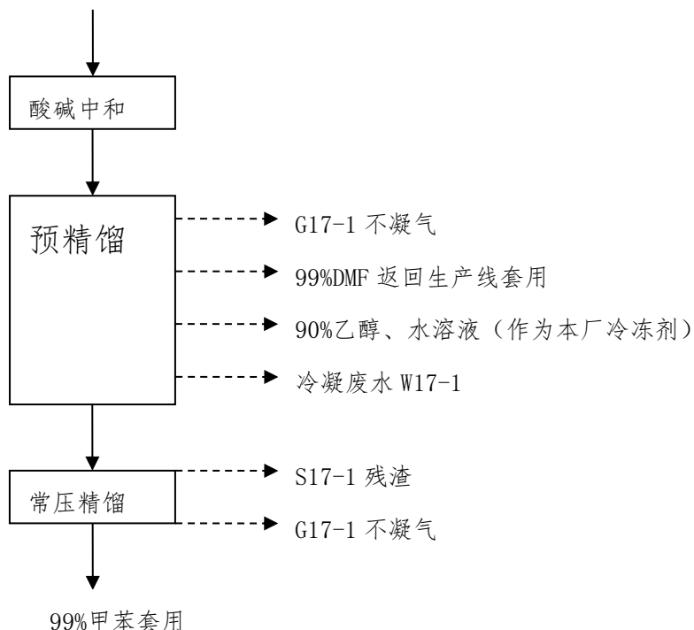
图 4.3-25 99%甲苯蒸馏提纯工艺流程图
