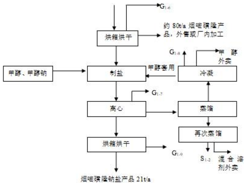
图 4.3-5 烟啉磷隆及其钠盐生产线工艺流程框图
